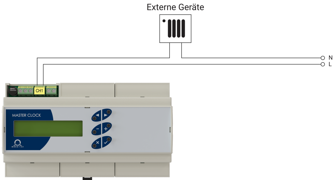
Anschluss von externen Geräten mit 230 VAC-Stromversorgung
