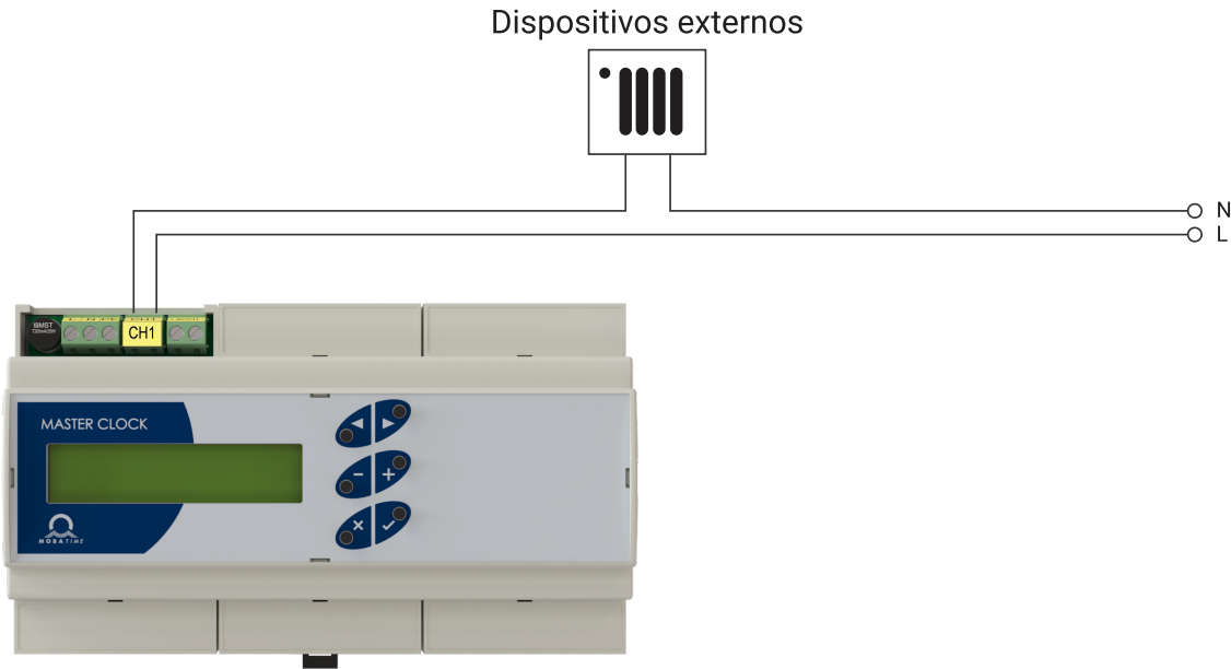
Conexión de dispositivos externos con alimentación de 230 VCA
