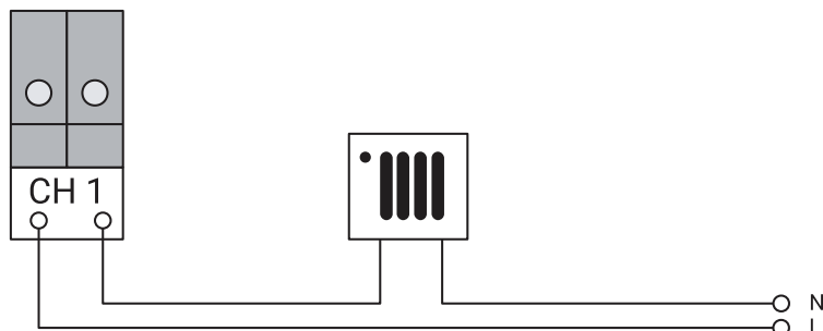
Připojení externích zařízení s napájením 230 VAC
