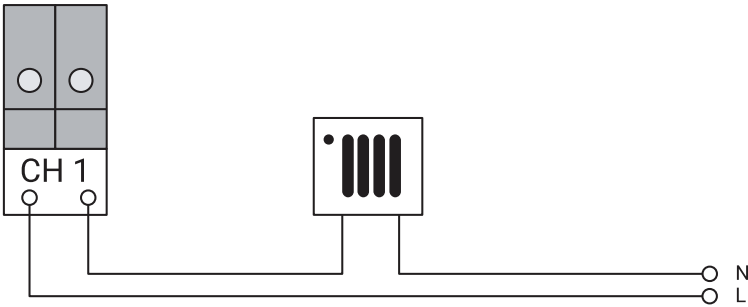
Connexion d'appareils externes avec une alimentation électrique de 230 VAC
