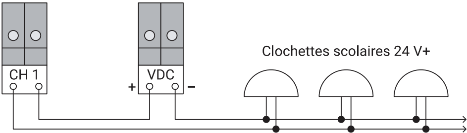
Raccordement des cloches de l'école
