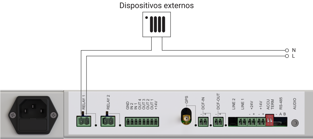
Conexión de dispositivos externos con alimentación de 230 VCA
