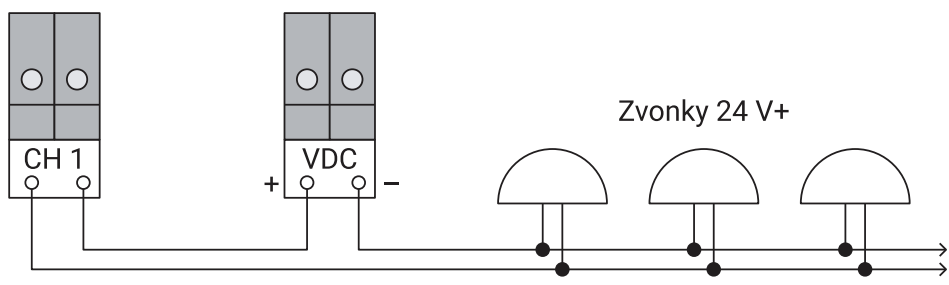
Připojení školních zvonků
