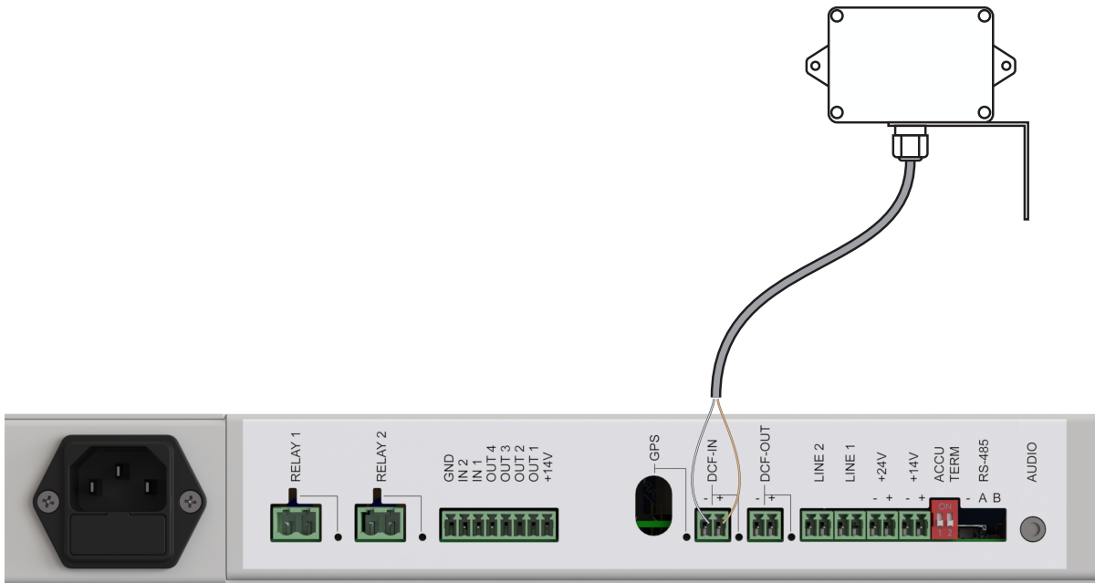
Tabulka barev drátů a připojení
