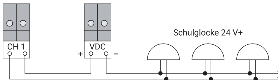
Anschluss von Schullocken
