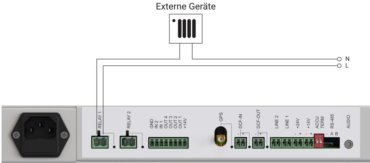
Anschluss von externen Geräten mit 230 VAC-Stromversorgung
