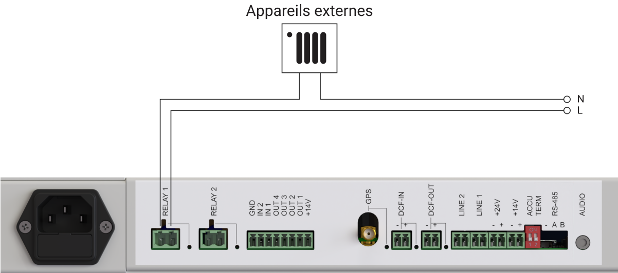
Connexion d'appareils externes avec une alimentation électrique de 230 VAC
