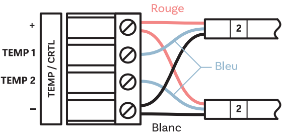
Bornier standard enfichable TEMP
