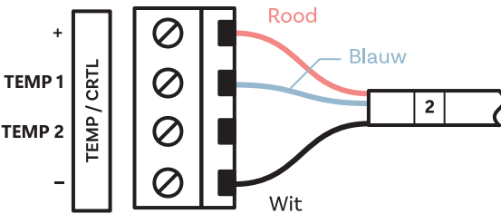
TEMP schroefklemmenblok (direct op printplaat digitale klok)
