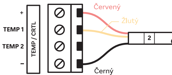
Šroubovací svorkovnice TEMP (přímo na desce plošných spojů digitálních hodin)
