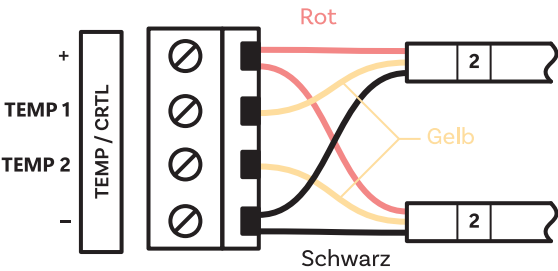
TEMP Schraubklemmenblock (direkt auf der Platine der Digitaluhr)
