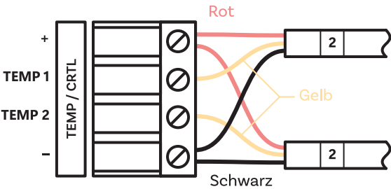
TEMP Steckbare Standard-Klemmenblock
