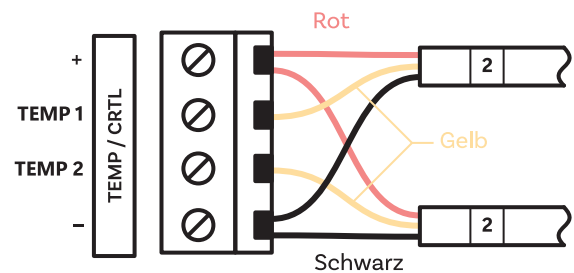
TEMP Schraubklemmenblock (direkt auf der Platine der Digitaluhr)
