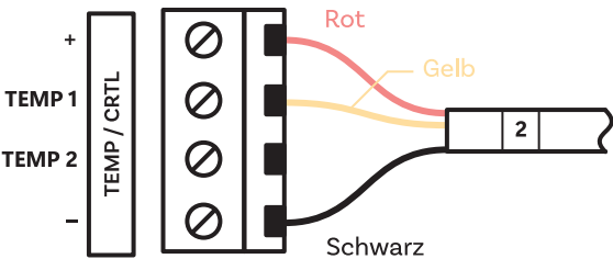
TEMP Schraubklemmenblock (direkt auf der Platine der Digitaluhr)
