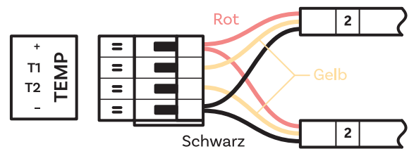
TEMP Steckbare Klemmenblock
