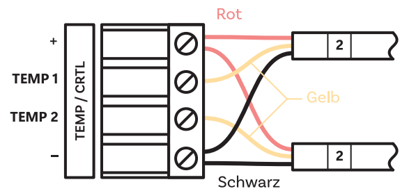
TEMP Steckbare Standard-Klemmenblock
