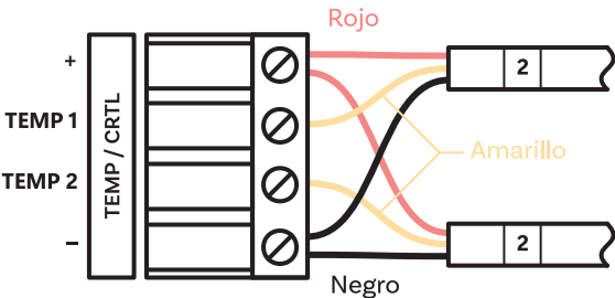
Bloque de terminales enchufable estándar TEMP
