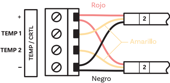
Bloque de terminales de tornillo TEMP (directamente en la placa de circuito impreso del reloj digital)
