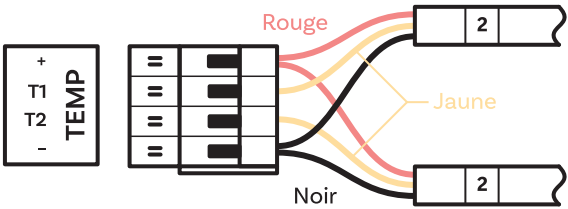
Bornier enfichable TEMP
