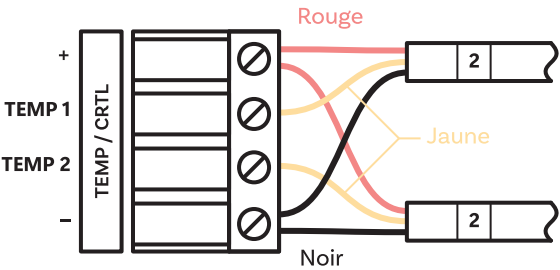
Bornier standard enfichable TEMP
