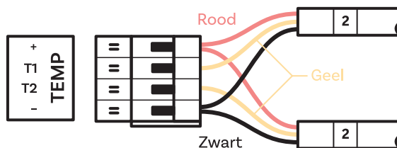
TEMP insteekklemmenblok
