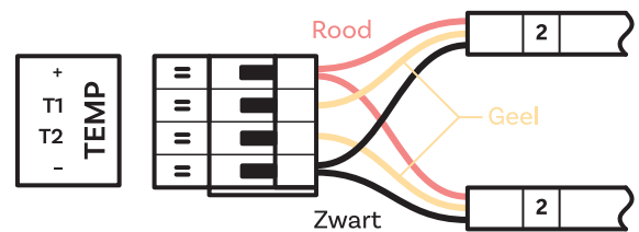
TEMP insteekklemmenblok
